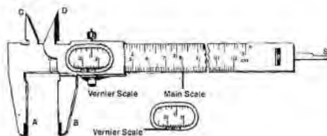
Vernier Callipers
